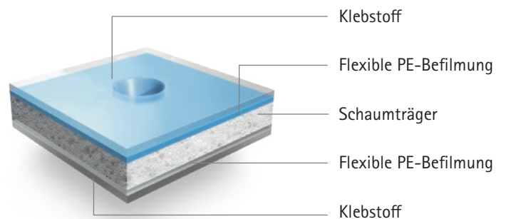
DuploFLEX® 5-Reihe mit beidseitiger, flexibler PE-Befilmung, die die einwirkenden Kräfte perfekt abfedert und Punktzuwachs verhindert.
