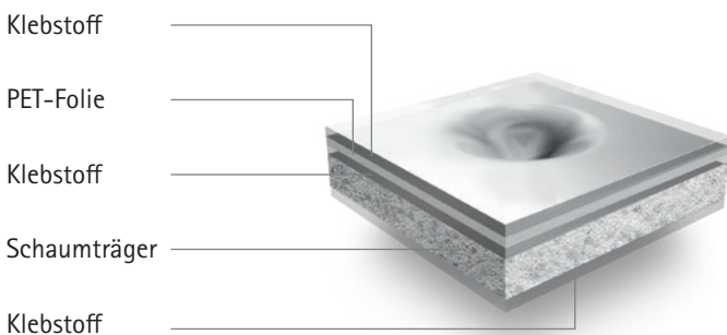
Herkömmliches Schaumklebeband mit kaschierter PET-Folie.
